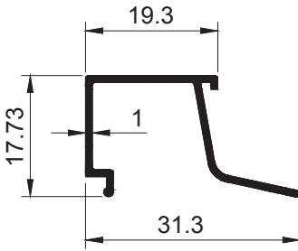
SECTION NO. - GL-120 EST. WEIGHT - 0.179 KG./M.
