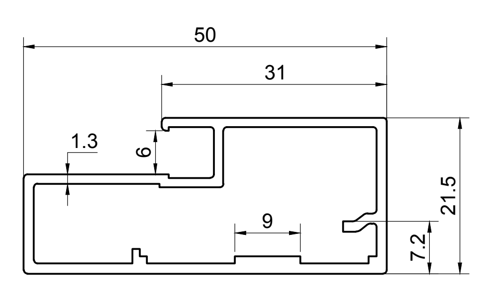
KCB-004 EST. WEIGHT 0.589 kg./m.
