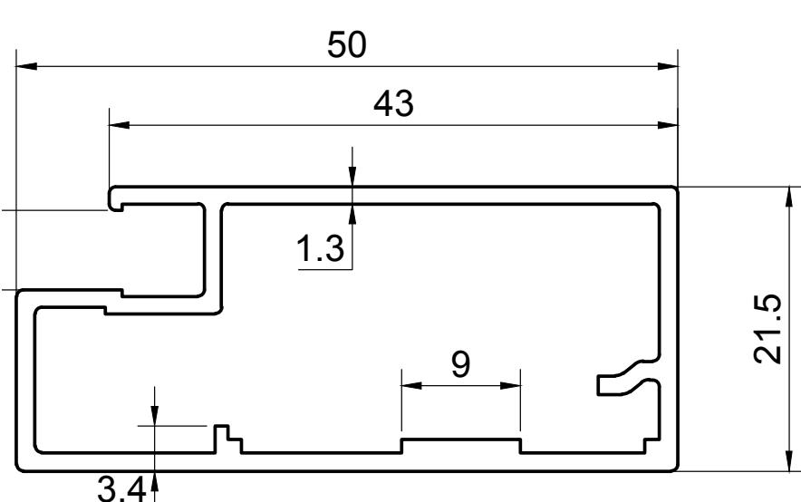
KCB-005 EST. WEIGHT 0.589 kg./m.
