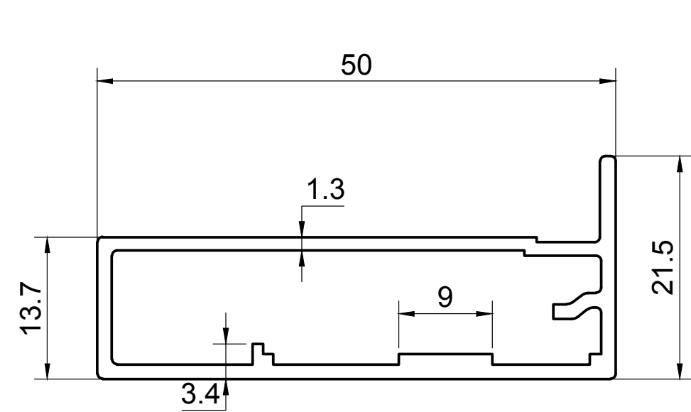
KCB-002 EST. WEIGHT 0.535 kg./m.
