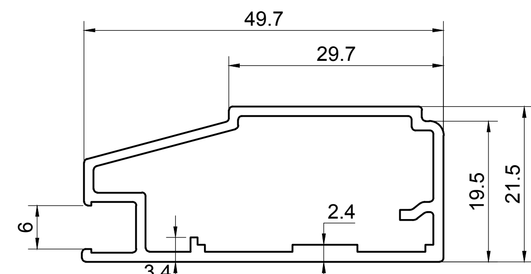
KCB-007 EST. WEIGHT 0.563 kg./m.
