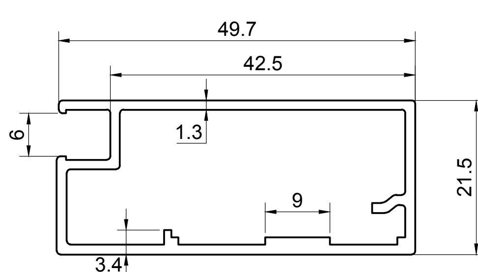
KCB-006 EST. WEIGHT 0.587 kg./m.
