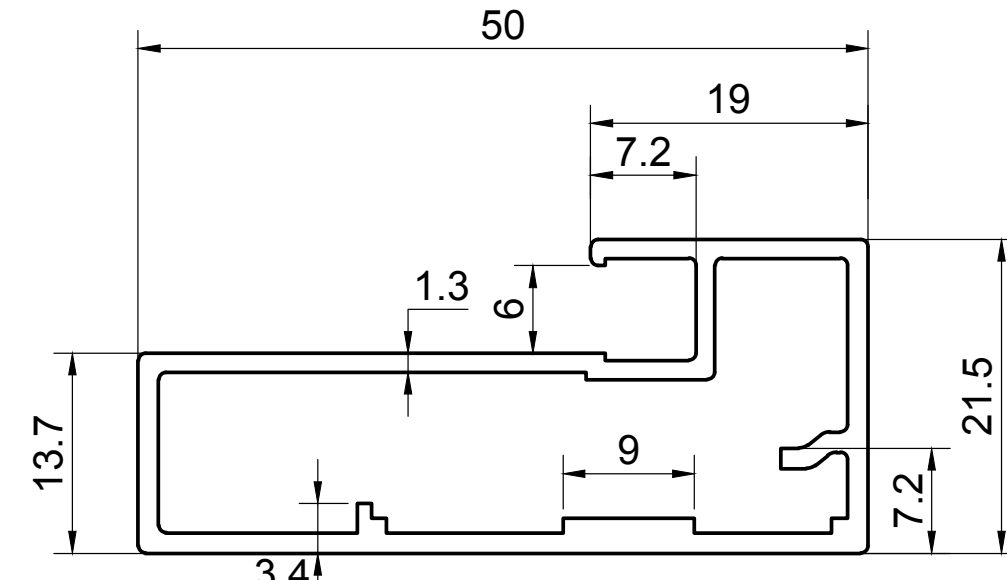
KCB-003 EST. WEIGHT 0.589 kg./m.
