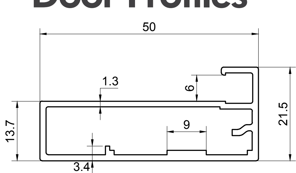
KCB-001 EST. WEIGHT 0.558 kg./m.
