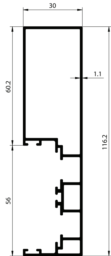
SECTION NO. - TSD-1201 EST. WEIGHT - 1.065 KG./M.
