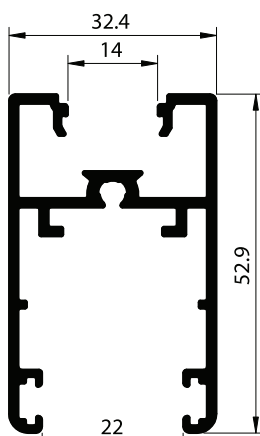
SECTION NO. - ESD-1506 EST. WEIGHT - 0.824 KG./M.
