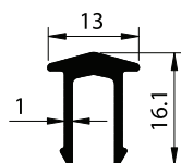
SECTION NO. - ESD-1003 EST. WEIGHT - 0.148 KG./M.
