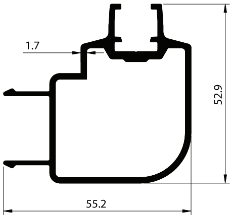
SECTION NO. - ESD-1903 EST. WEIGHT - 1.004 KG./M.
