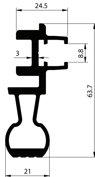
SECTION NO. - ESD-1902 EST. WEIGHT - 1.194 KG./M.
