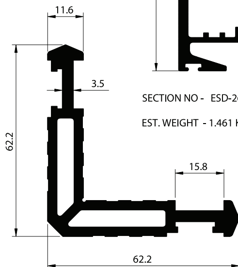
SECTION NO. - ABS-SD10 EST. WEIGHT - 1.825 KG./M.
