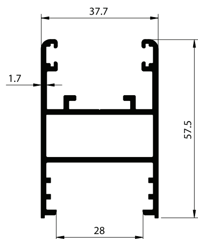
SECTION NO - ESD-2701 EST. WEIGHT - 10.933 KG./M
