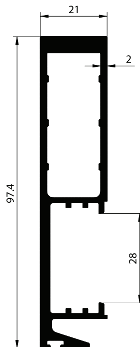
SECTION NO - ESD-2601 EST. WEIGHT - 1.461 KG./M
