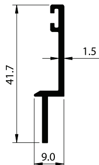
SECTION NO. - ESD-1302 EST. WEIGHT - 0.218 KG./M.
