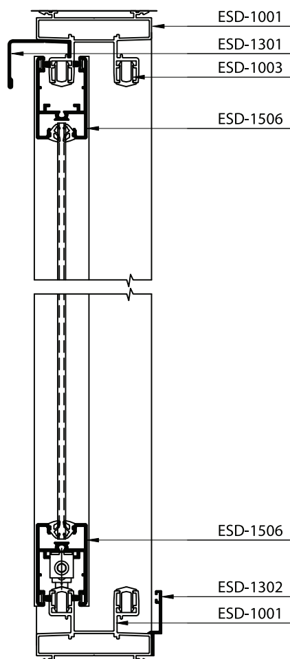
SECTION :- A-A
