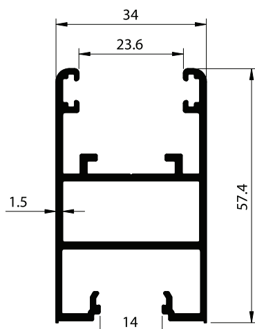
SECTION NO. - ESD-1701 EST. WEIGHT - 0.920 KG./M.
