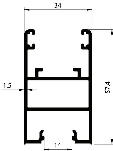
SECTION NO. - ESD-1701 EST. WEIGHT - 0.920 KG./M.
