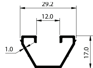
SECTION NO - ESD-2902 EST. WEIGHT - 0.191 KG./M
