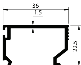
SECTION NO. - GL-108 EST. WEIGHT - 0.357 KG./M.
