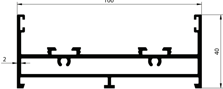
SECTION NO. - SDG-2002 EST. WEIGHT - 1.109 KG./M.
