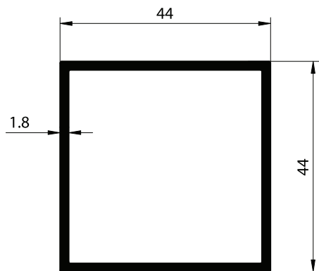
SECTION NO. - P-1119 EST. WEIGHT - 0.820 KG./M.
