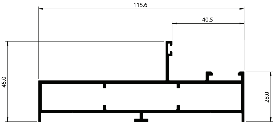
SECTION NO. - ECA-26 EST. WEIGHT - 1.414 KG./M.
