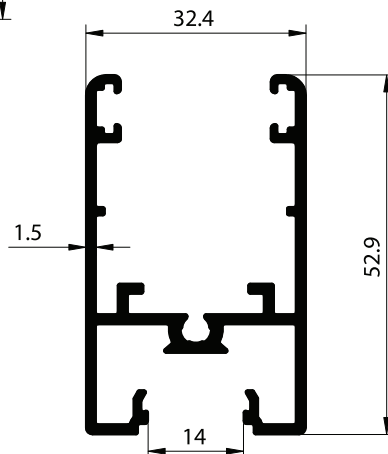
SECTION NO. - ESD-1506 EST. WEIGHT - 0.824 KG./M.
