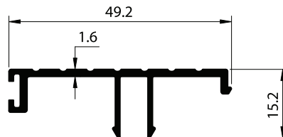
SECTION NO - ESD-2302 EST. WEIGHT - 0.334 KG./M
