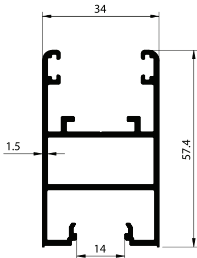
SECTION NO. - ESD-1701 EST. WEIGHT - 0.920 KG./M.
