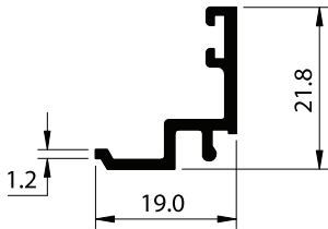
SECTION NO - GL-123 EST. WEIGHT - 0.187 KG./M GLASS GAP - 36.5 MM
