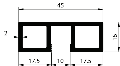
SECTION NO. - TSD-1701 EST. WEIGHT - 0.695 KG./M.
