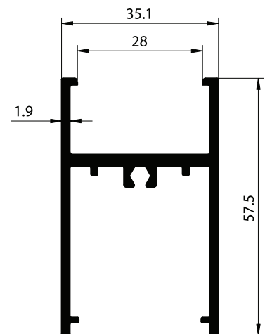
SECTION NO - ESD-2508 EST. WEIGHT - 0.895 KG./M
