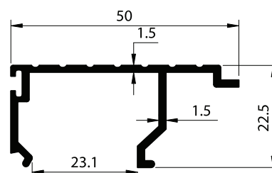
SECTION NO. - GL-109 EST. WEIGHT - 0.408
