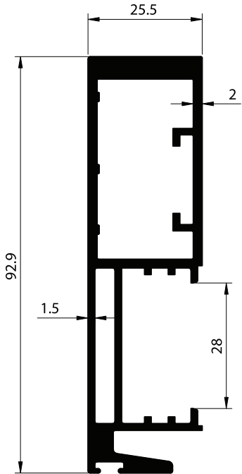
SECTION NO. - UTS-1601 EST. WEIGHT - 1.640 KG./M.
