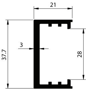
SECTION NO. - UTS-1501 EST. WEIGHT - 0.472 KG./M.
