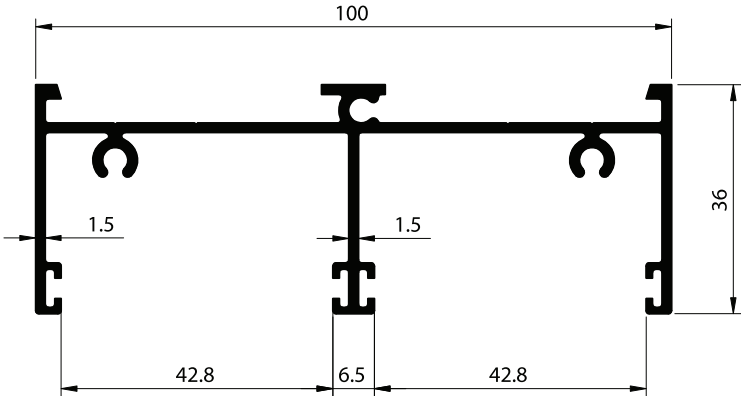
SECTION NO. - SDG-2002 EST. WEIGHT - 1.109 KG./M.
