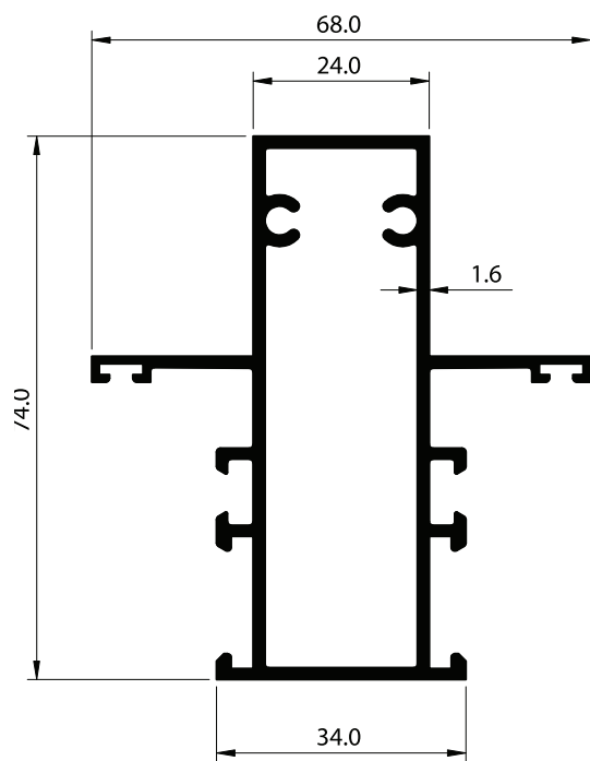
SECTION NO. - ECA-28 EST. WEIGHT - 1.290 KG./M.
