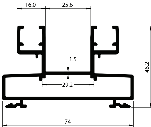
SECTION NO. - ESD-1001 EST. WEIGHT - 1.445 KG./M.
