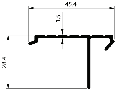
SECTION NO. - SD-1302 EST. WEIGHT - 0.303 KG./M.
