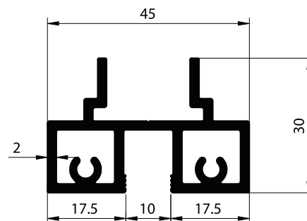
SECTION NO. - TSD-1401 EST. WEIGHT - 0.992 KG./M.
