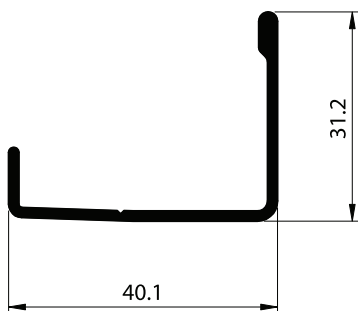
SECTION NO. - ESD-1301 EST. WEIGHT - 0.332 KG./M.
