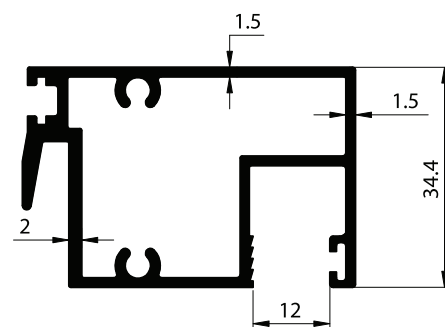
SECTION NO. - ESD-3602 EST. WEIGHT - 0.985 KG./M.
