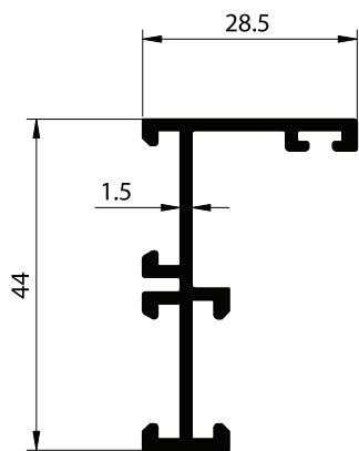
SECTION NO. - EPT-003 EST. WEIGHT - 0.481 KG./M.
