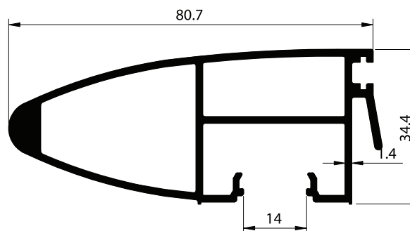
EST. WEIGHT - 1.165 SECTION NO - ESD-3601
