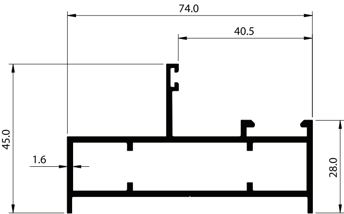
SECTION NO. - ECA-23 EST. WEIGHT - 1.007 KG./M.
