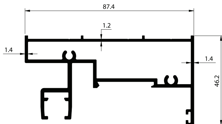
SECTION NO. - ESD-3002 EST. WEIGHT - 1.344 KG./M.
