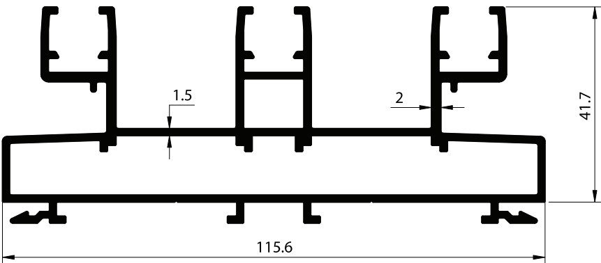
SECTION NO. - ESD-1002 EST. WEIGHT - 2.184 KG./M.
