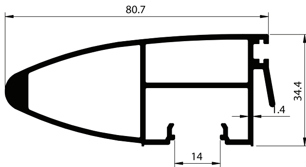
EST. WEIGHT - 1.165 SECTION NO - ESD-3601
