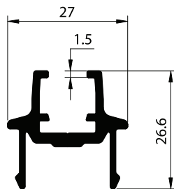
SECTION NO. - ESD-1901 EST. WEIGHT - 0.438 KG./M.
