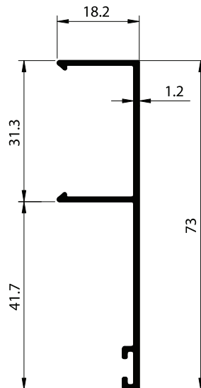
SECTION NO. - TSD-1002 EST. WEIGHT - 0.356 KG./M.
