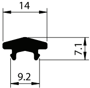
SECTION NO. - ABS-SD07 EST. WEIGHT - 0.138 KG./M.
