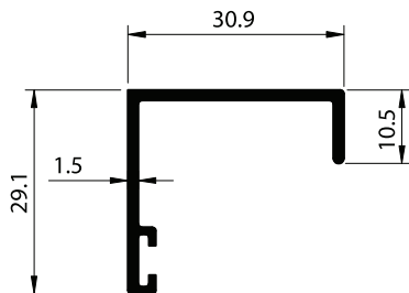
SECTION NO - ESD-2301 EST. WEIGHT - 0.295 KG./M
