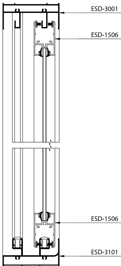
SECTION :- A-A
