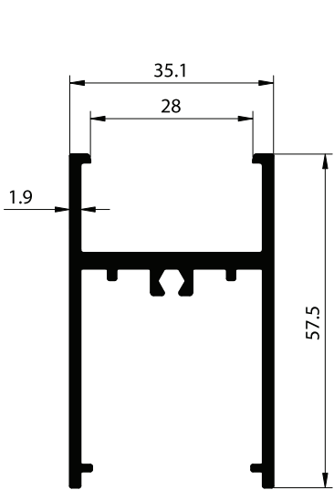
SECTION NO - ESD-2508 EST. WEIGHT - 0.895 KG./M
