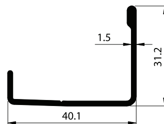
SECTION NO. - ESD-1301 EST. WEIGHT - 0.332 KG./M.
