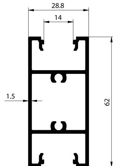
SECTION NO. - ESD-1801 EST. WEIGHT - 0.956 KG./M.
