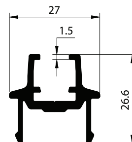
SECTION NO. - ESD-1901 EST. WEIGHT - 0.438 KG./M.
