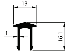
SECTION NO. - ESD-1003 EST. WEIGHT - 0.148 KG./M.
